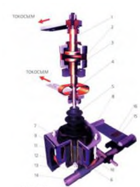
Рис.2 Конструкция полюса выключателя
