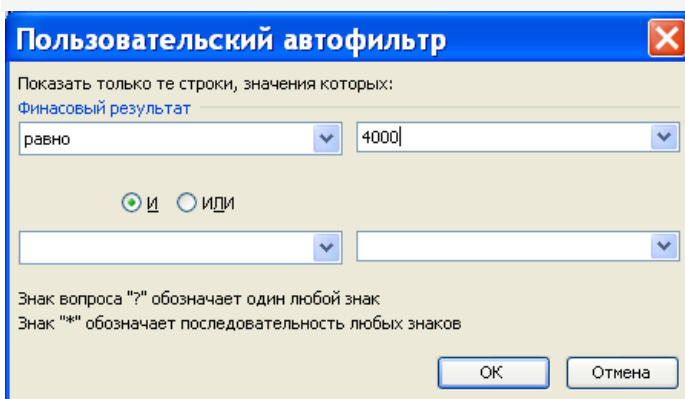
Рис.1.6. Пользовательский автофильтр
