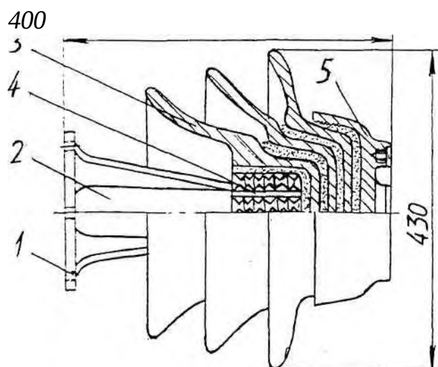
Рис 2. Опорно - штыревой изолятор.
