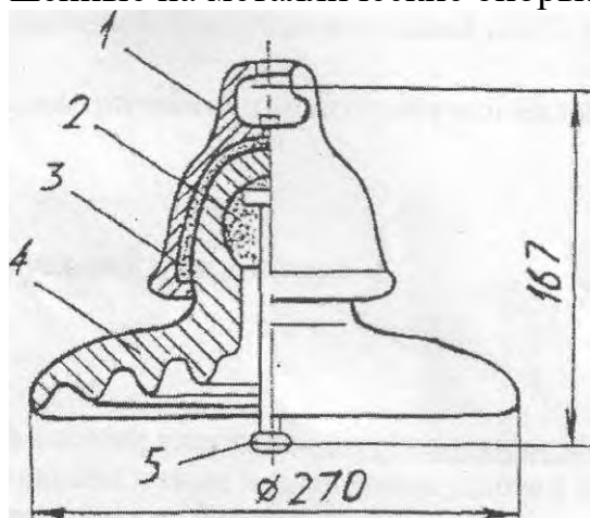
Рис. 5 Подвесной изолятор
