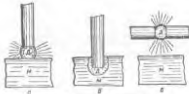
Рис. 20. Разновидности дуговых печей
