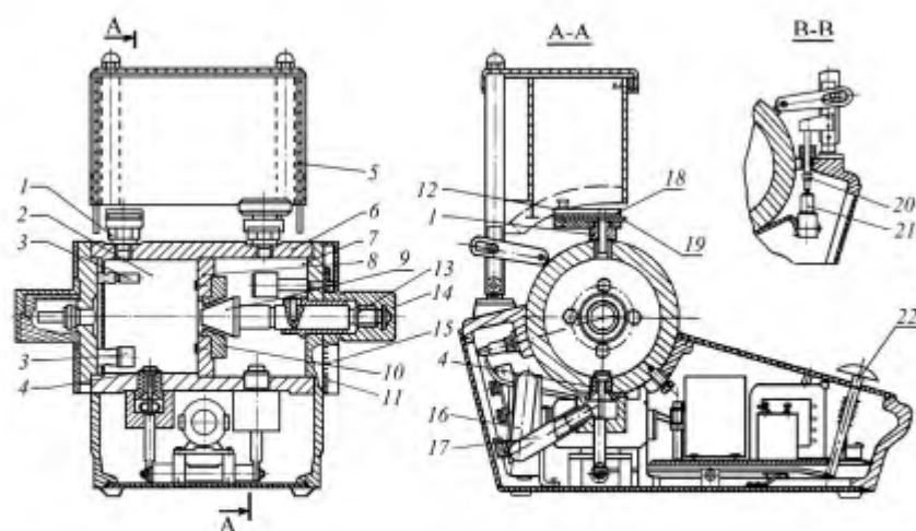
Рис. 13.3. Устройство стенда ОТ 17 для определения величины тушащего зазора:
