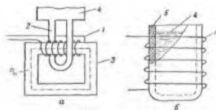
Рис. 23. Принципиальные схемы индукционного нагрева: а — схема печи с железным сердечником; б — схема печи без сердечника; 1 — первичная обмотка (индуктор); 2 — канал, выполненный из металла; 3 — железный сердечник; 4 — металлическая заготовка; 5 — футеровка печи (углерод)
