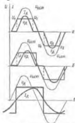
Рис. 21 Кривые мгновенного значения силы тока I_d , напряжения дуги U_d и напряжения питающего источника U_{ист} : а — индуктивное сопротивление цепи; б — горение дуги прерывистой; в — непрерывное горение дуги при индуктивном сопротивлении; г — горение дуги прерывистой; д — горение дуги прерывистой; е — горение дуги непрерывной.
