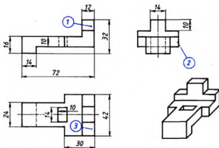
Рис. 148. Упор
