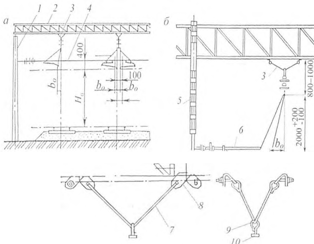
Рис. 1.5. Крепление несущего троса на жесткой поперечине: а - общий вид с фиксирующим тросом; б - с фиксаторной стойкой; в - тре-угольный подвес со скобами: 1 - опора; 2 - поперечина (ригель); 3 - тре-угольный подвес; 4- трос фиксирующий; 5- стойка фиксаторная; 6 - фиксатор; 7- штанга диаметром 12 мм; 8 - скоба; 9 - серьга с пестиком; 10 - болт крюковой
