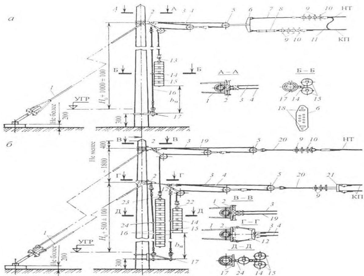
Рис. 1.1. Анкеровка компенсированной цепной контактной подвески переменного (а) и постоянного (б) тока:
