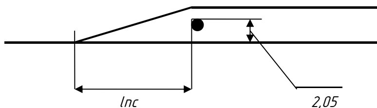
Рисунок 1 Схема установки предельного столбика в междупутье
