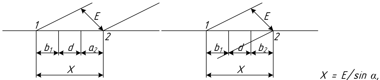
Рисунок 6 Схемы взаимного расположения двух стрелочных переводов.
