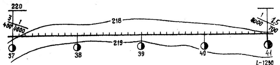
План местности в горизонталях №2
