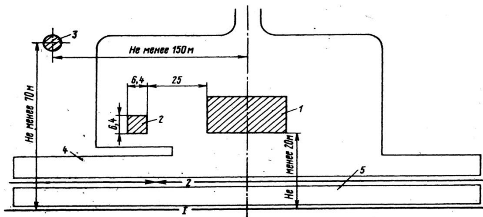
Рисунок 8 Схема размещения пассажирских устройств на промежуточной станции: 1 - пассажирское здание, 2 - блок вспомогательных помещений, 3 - водоемное здание, 4 - основная пассажирская платформа, 5 - промежуточная пассажирская платформа.
