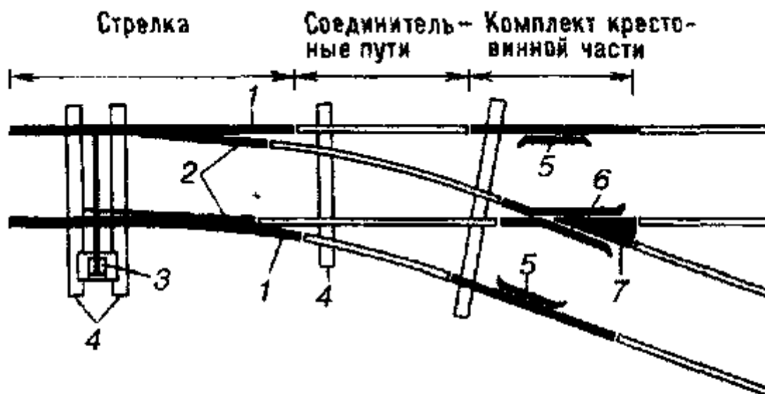
Рис. 4.78. Схема одиночного стрелочного перевода: 1 – рамные рельсы; 2 – остряки; 3 – переводной механизм; 4 – переводные бруссы; 5 – контррельсы; 6 – усовик; 7 – сердечник
