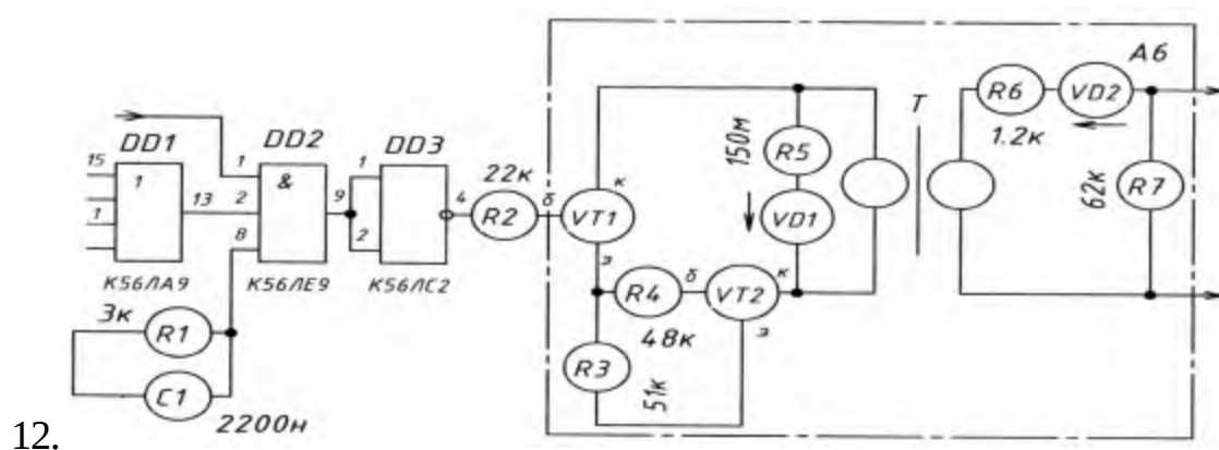
Схема питания рабочих цепей стрелочных электроприводов панели типа ПР-ЭЦ25 (фрагмент силовой установки)
