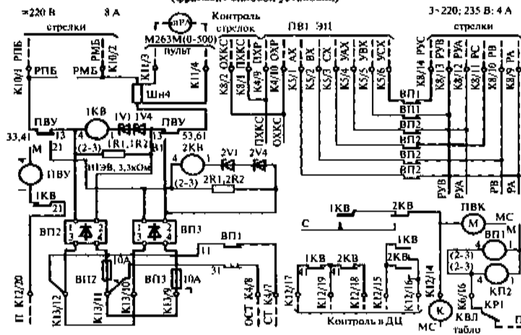
Схема питания рабочих цепей стрелочных электроприводов модели типа ПР-ЭЦ25 (фрагмент силовой установки)
