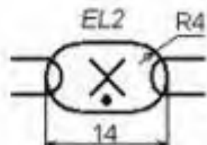
Газоразрядная (люминисцентная)
