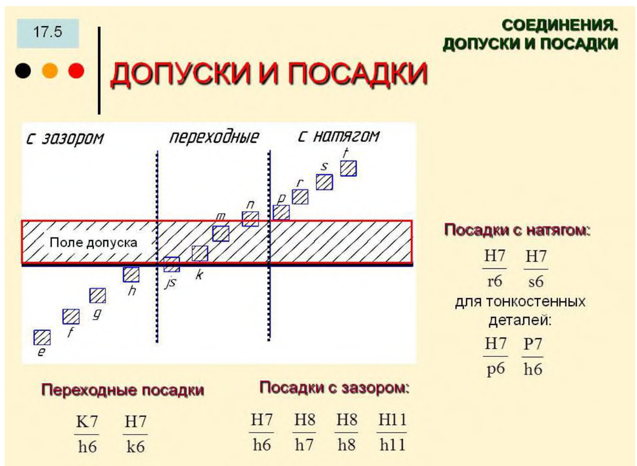
Рисунок 13. Примеры размещения полей допуска вала и отверстия в системе «отверстие».
