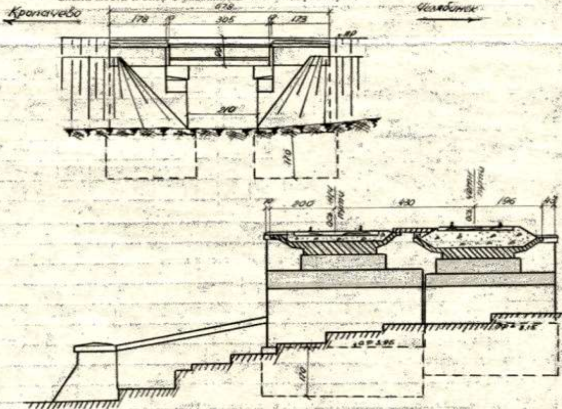
Схема моста и опор с указанием основных размеров:
