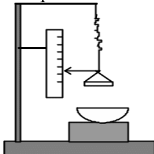
Рис. 1. Схема установки
