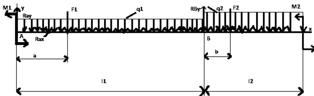
Рис. 6. Расчетная схема балки.
