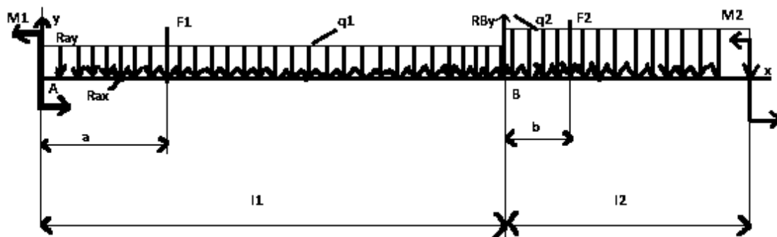
Рис. 6. Расчетная схема балки.
