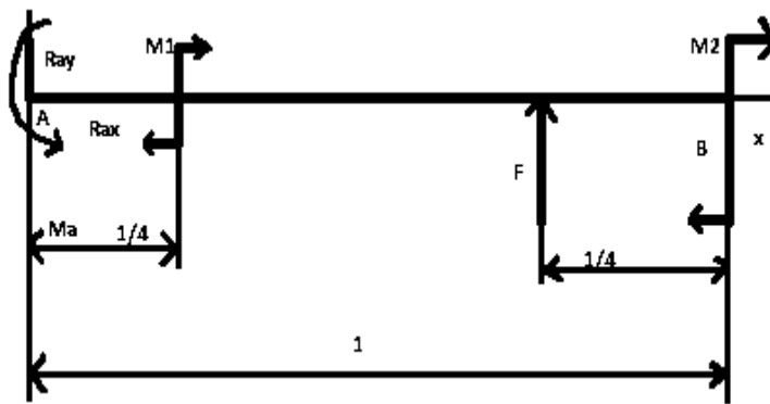
Рис. 7. Схема балки с жесткой заделкой
