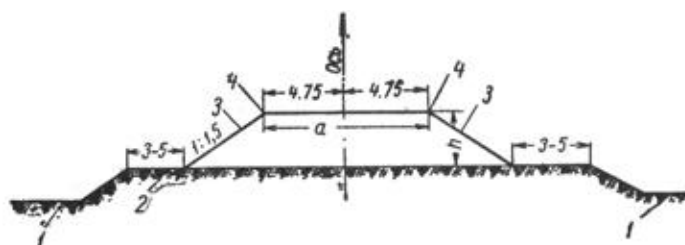
Рис. 1. Поперечный профиль насыпи 1 — резерв; 2 — берма; 3 — линия откоса; 4 — бровка; а — ширина насыпи; h — высота насыпи
