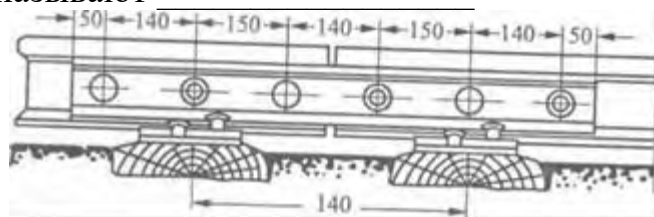
Рис. 2. Боковой вид стыка
