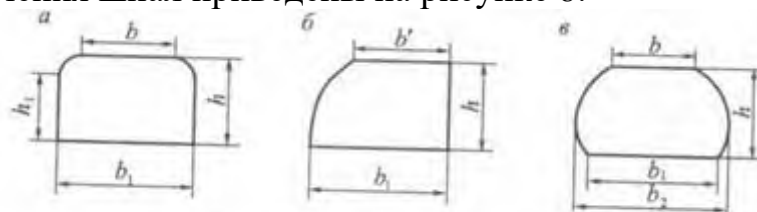
Рис. 8. Поперечное сечение шпал
