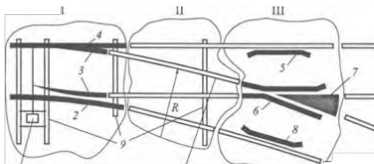
Рис.1. Обыкновенный стрелочный перевод
