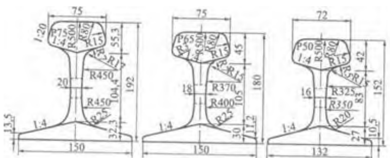
Рис. 1. Основные типы рельсов
