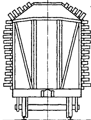
Рисунок 5 – Габаритная рама
