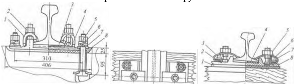
Рис. 4. Скрепление КБ-65 с прутковой клеммой
