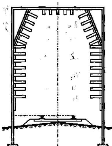
Рисунок 6 – Габаритные ворота
