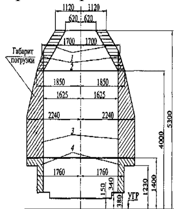
Рисунок 4 – Габарит погрузки
