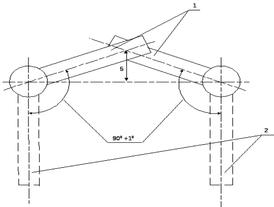
Рисунок 9.1. Положение контактных ножей разъединителя типа РЛНД-35/1000
