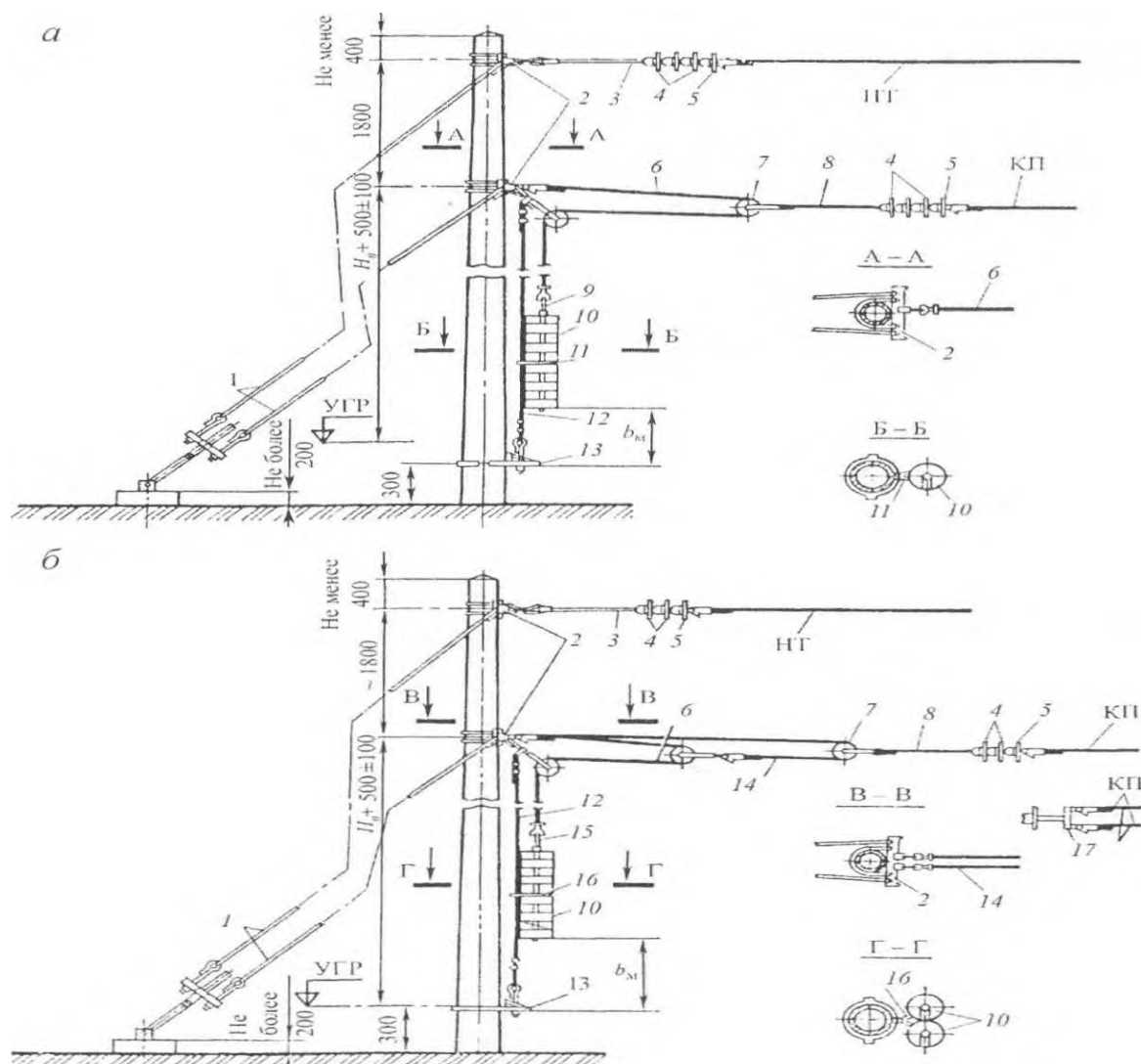
Рис. 1.2. Анкеровка полукомпенсированной цепной подвески переменного тока с двухблочным компенсатором (а) и постоянного тока с трехблочным компенсатором (б):
