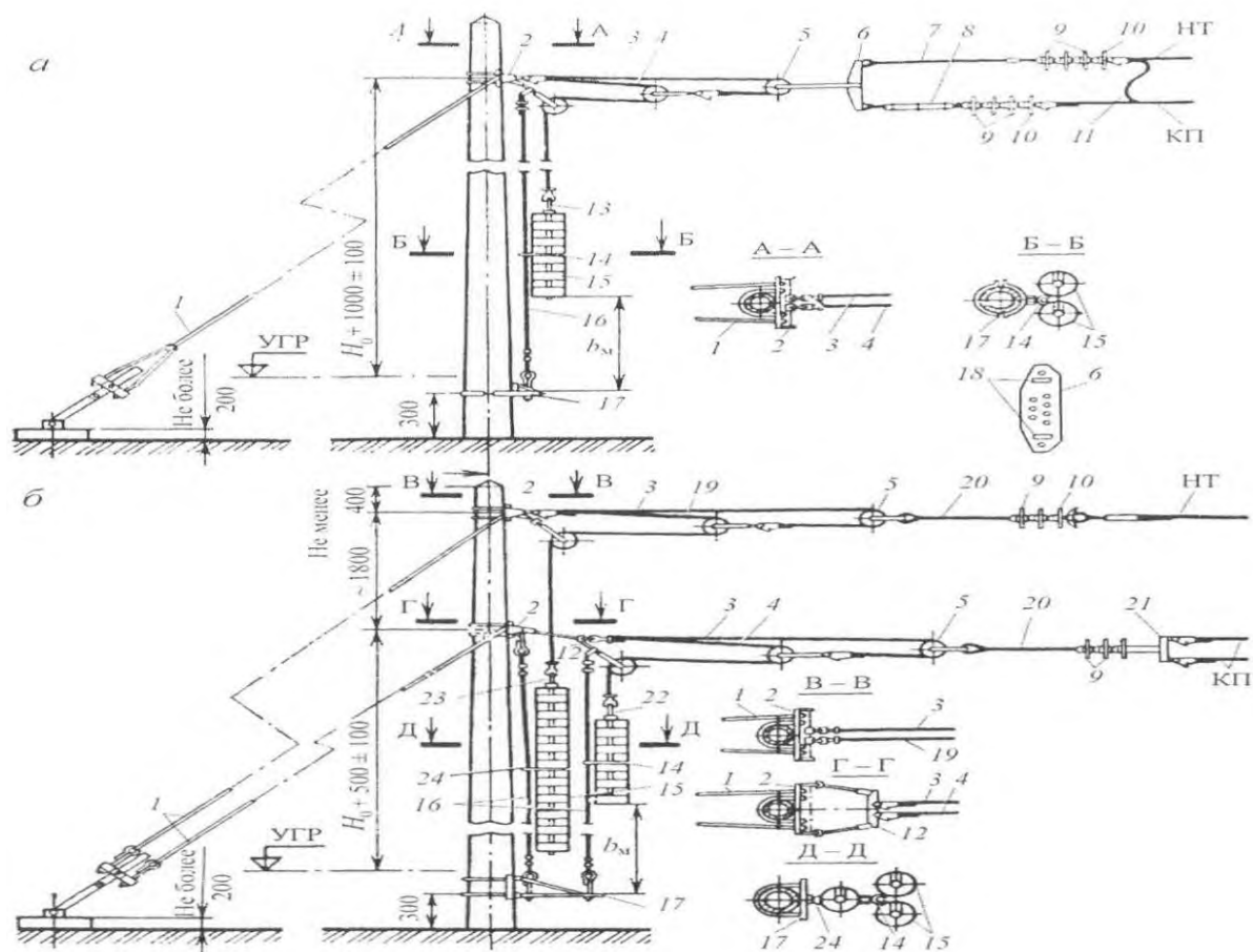
Рис. 1.1. Анкеровка компенсированной цепной контактной подвески переменного (я) и постоянного (б) тока:
