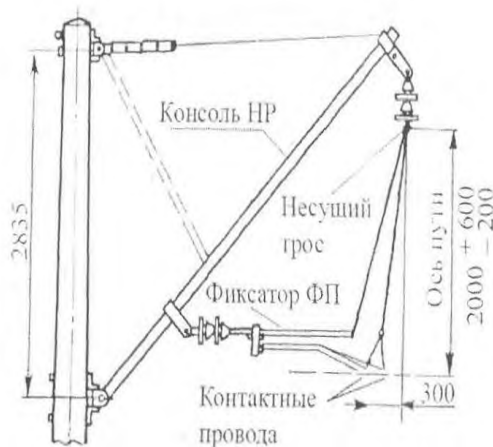
Рис. 1.4. Крепление несущего троса на неизолированной консоли
