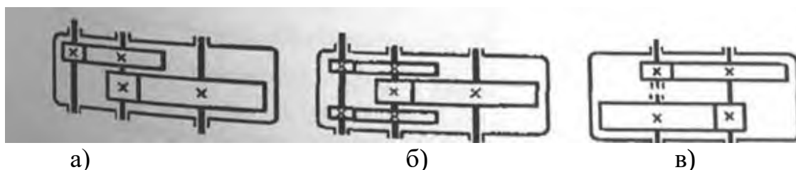
Рисунок 1 – Кинематические схемы цилиндрических двухступенчатых редукторов
