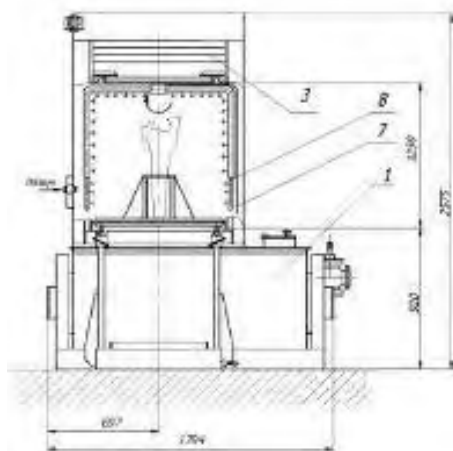
Рисунок 8.1 - Машина для мойки корпусов автосцепки
