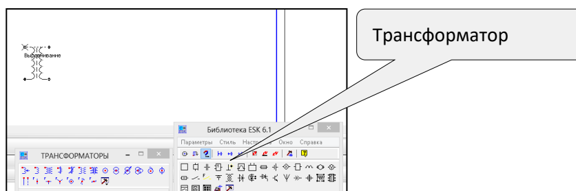
Рисунок 10.5 – Выполнение трансформатора
