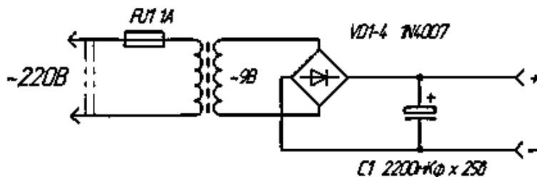
Рисунок 10.1 – Схема блока питания
